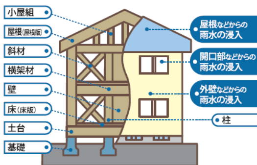
保険のお支払い対象となる基本構造部分のイメージ図
